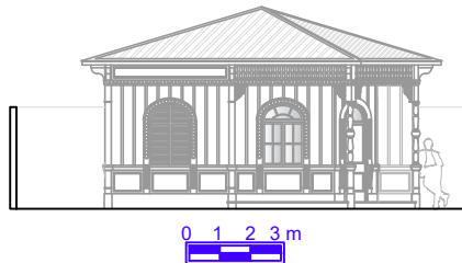
Elevation 01
